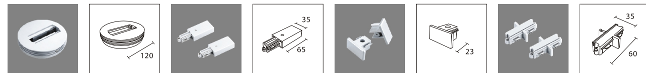
HT-101N Monopoint 230V · 16A Max load: 20N HT-L01(L/R) Live end 230V · 16A HT-ECAP End Cover HT-J01 Mini straight connetors 230V · 16A
