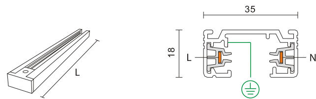
HT-1M · 2M · 3M 1-Circuit HT Series(Surface Mounted) 220V · 16A
